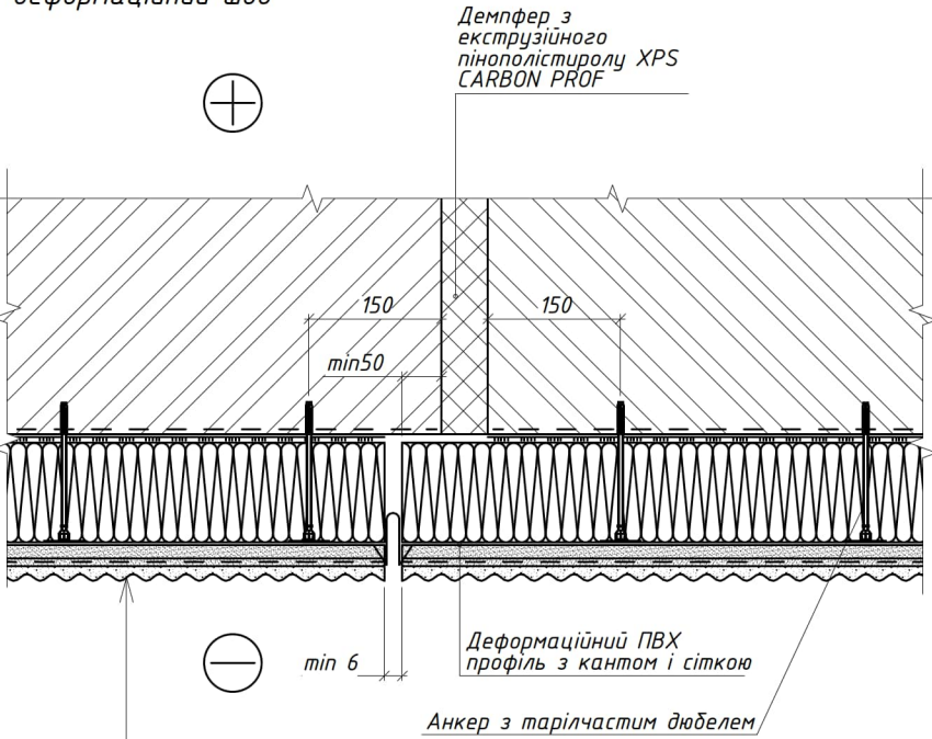
Вузол М міжсекційний деформаційний шов
