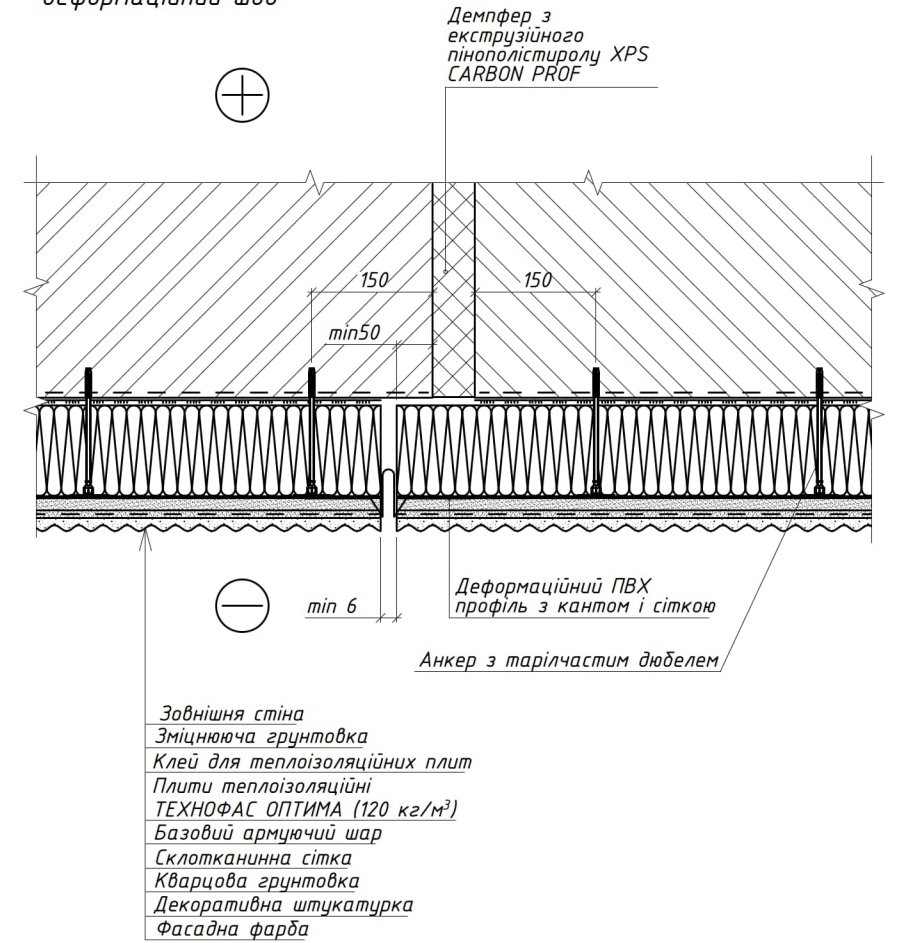
Вузол М міжсекційний деформаційний шов
