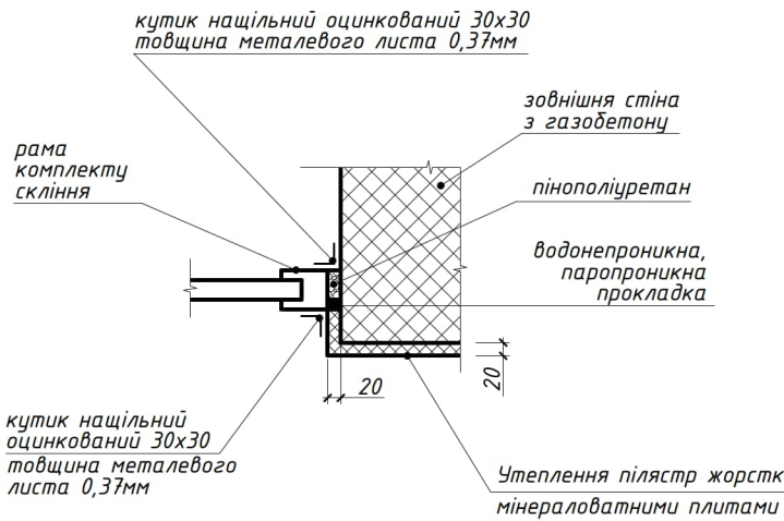
Вузол Б типовий вузол вертикального примикання комплектів скління
