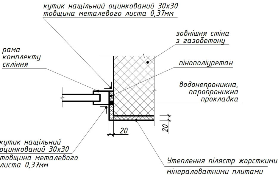
Вузол Б типовий вузол вертикального примикання комплектів скління
