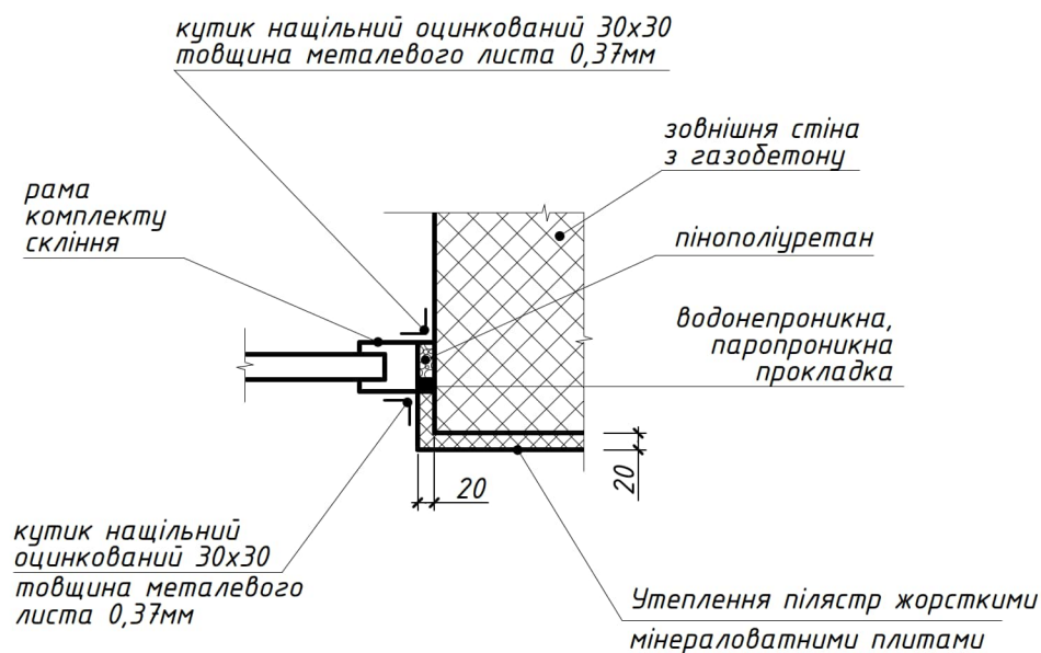
Вузол Б
