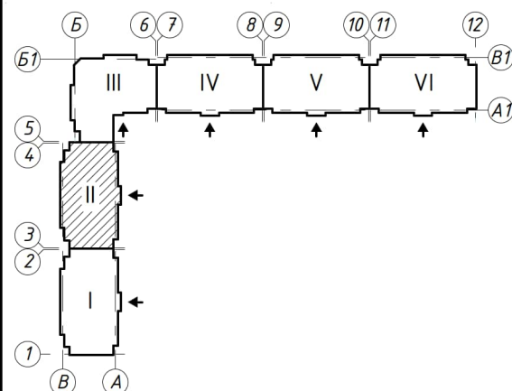
Блок-схема секцій
