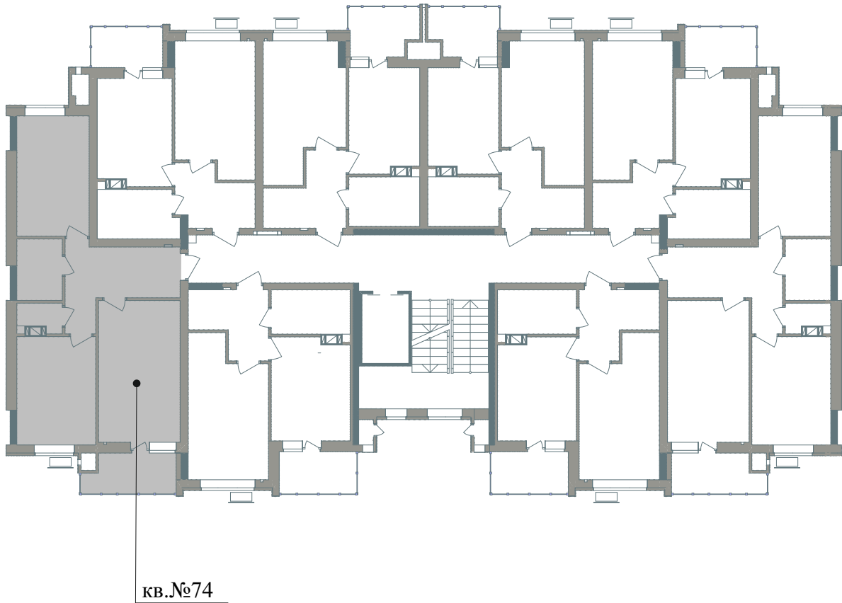
Схема розміщення МОН - №74 на поверсі
