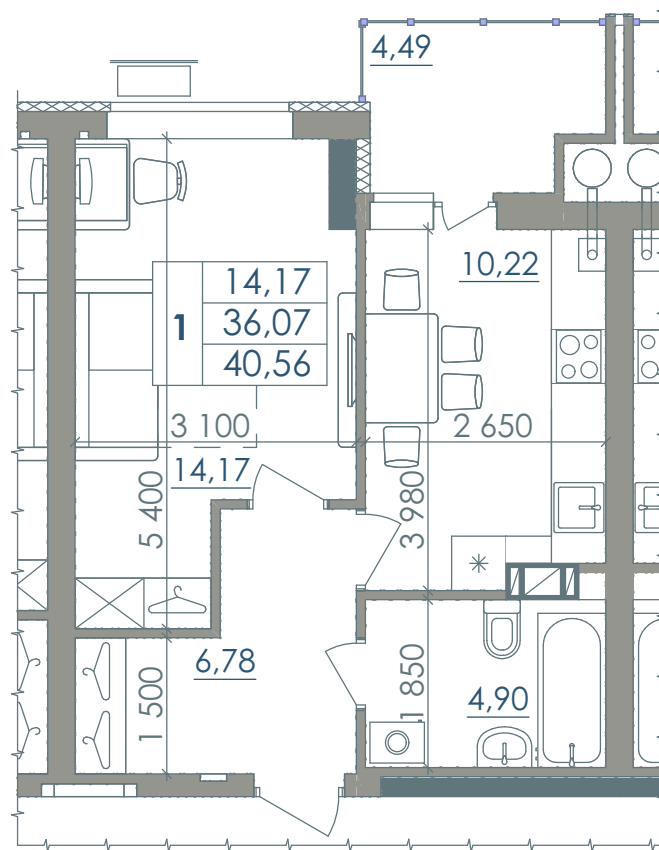
Графічне зображення схеми будівельного плану МОН - №212
