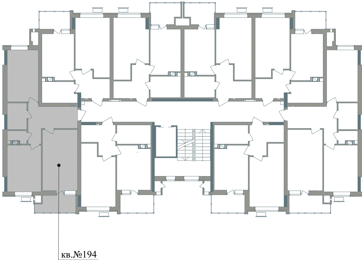
Схема розміщення МОН - №194 на поверсі
