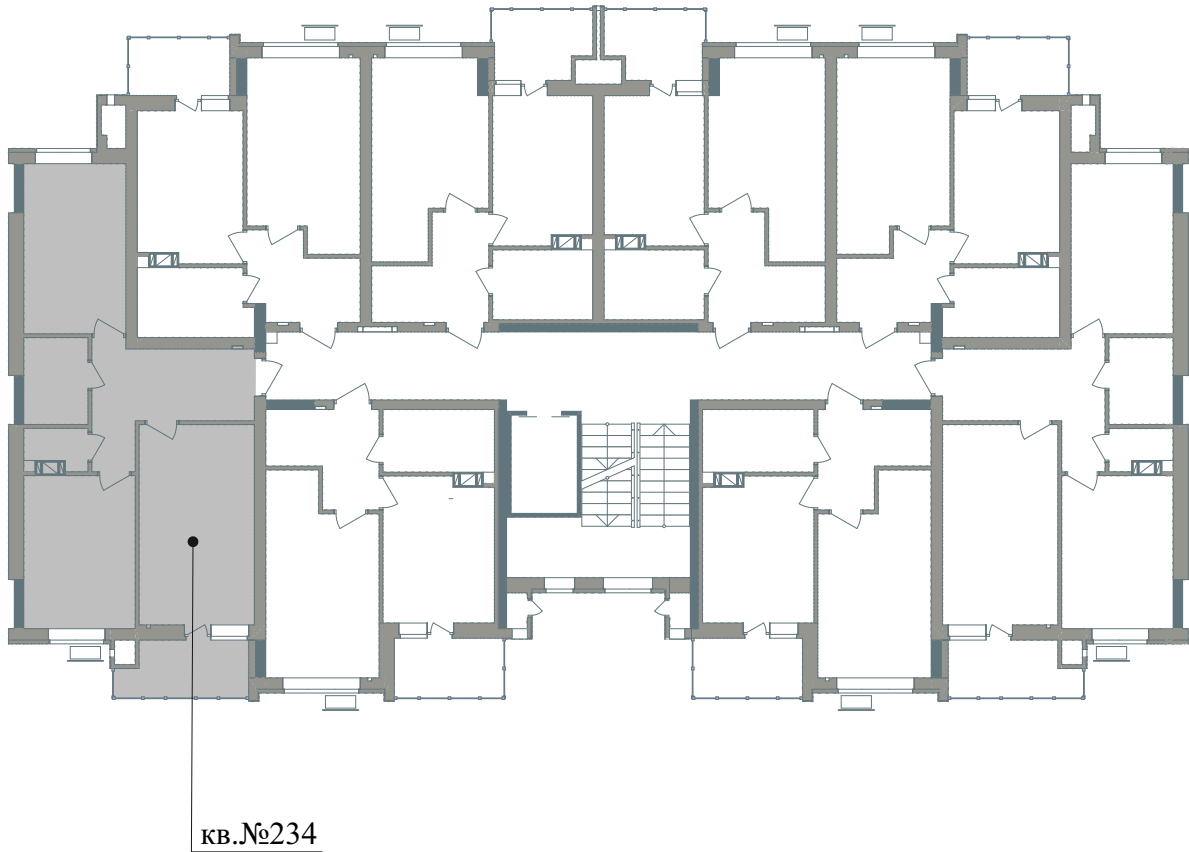
Схема розміщення МОН - №234 на поверсі
