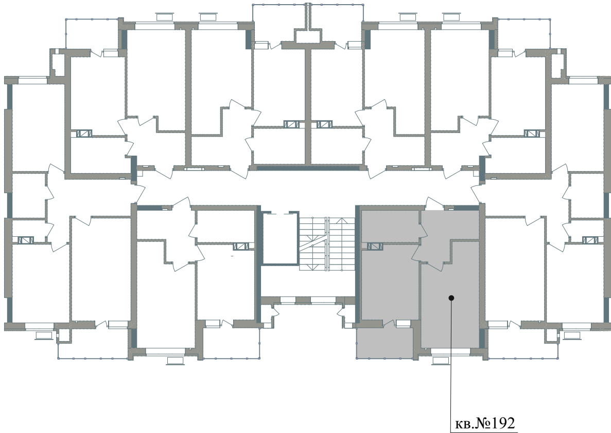
Схема розміщення МОН - №192 на поверсі
