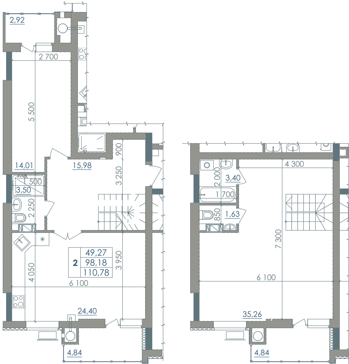
Графічне зображення схеми будівельного плану МОН - №242
