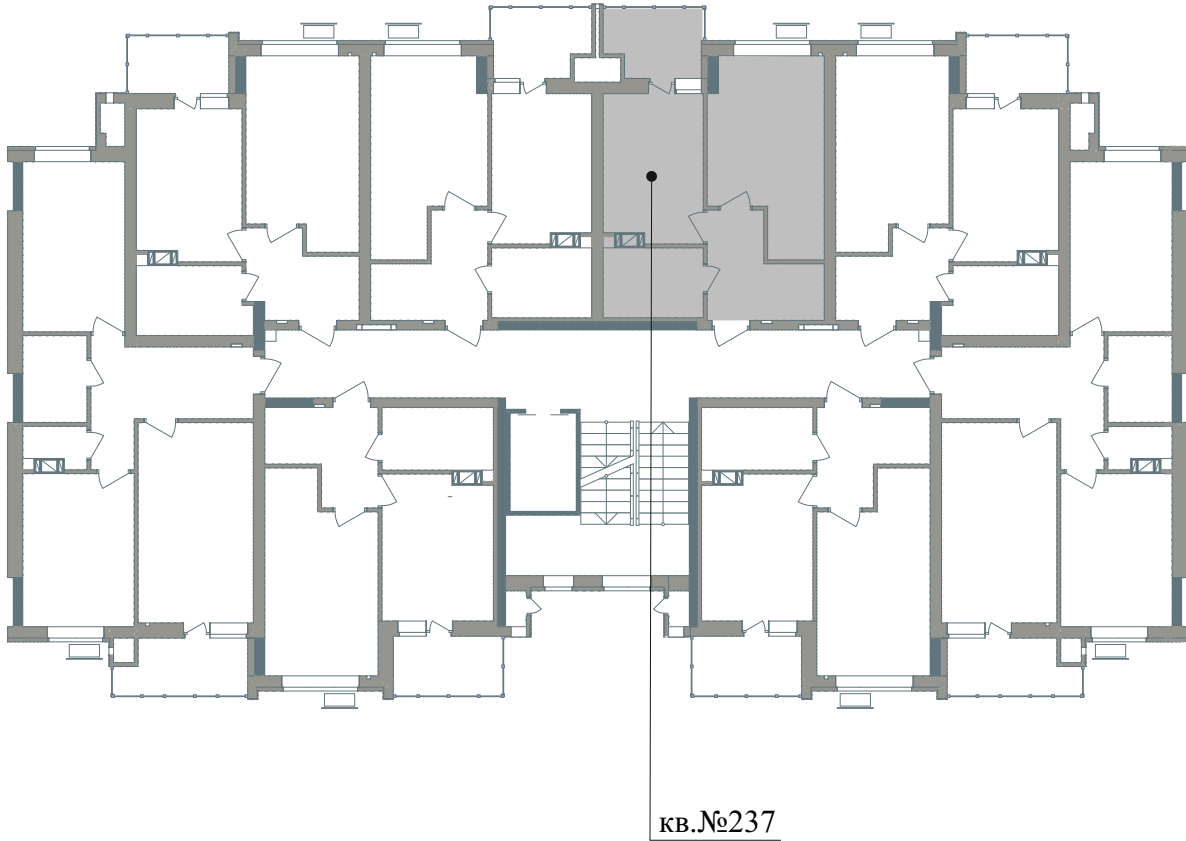
Схема розміщення МОН - №237 на поверсі
