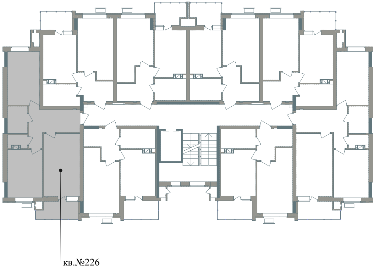
Схема розміщення МОН - №226 на поверсі
