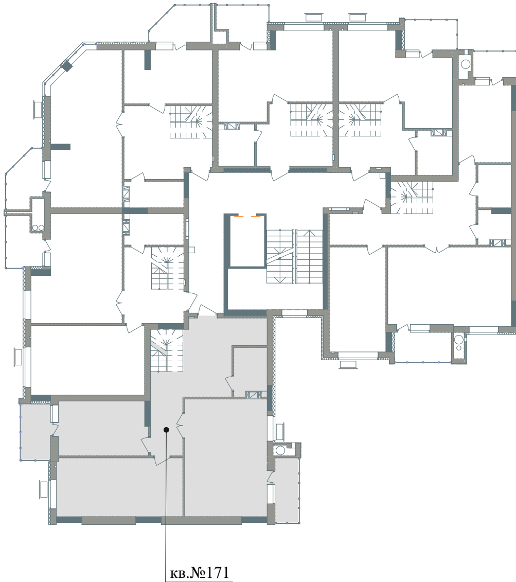
Схема розміщення МОН - №171 на поверсі
