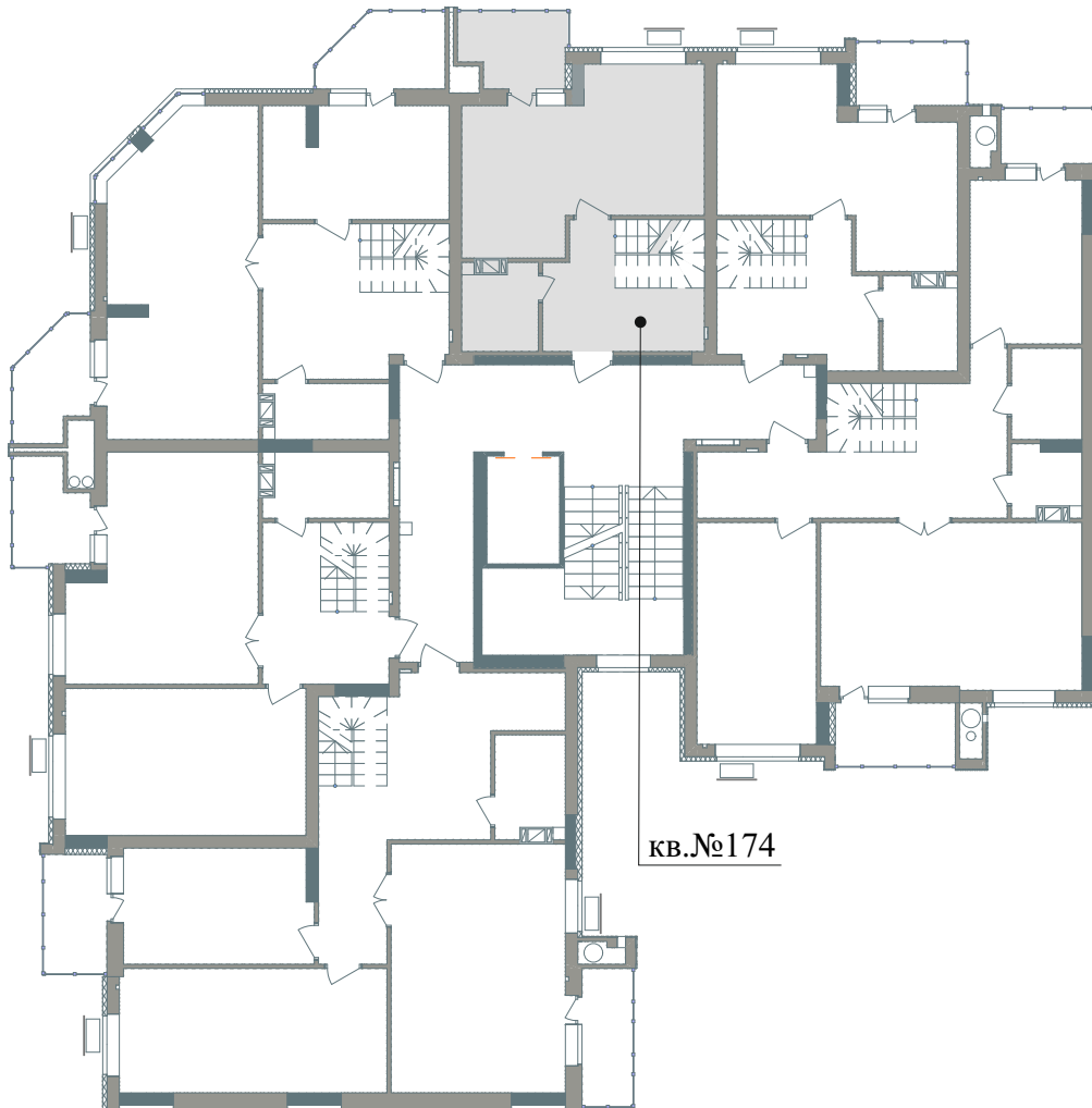
Схема розміщення МОН - №174 на поверсі
