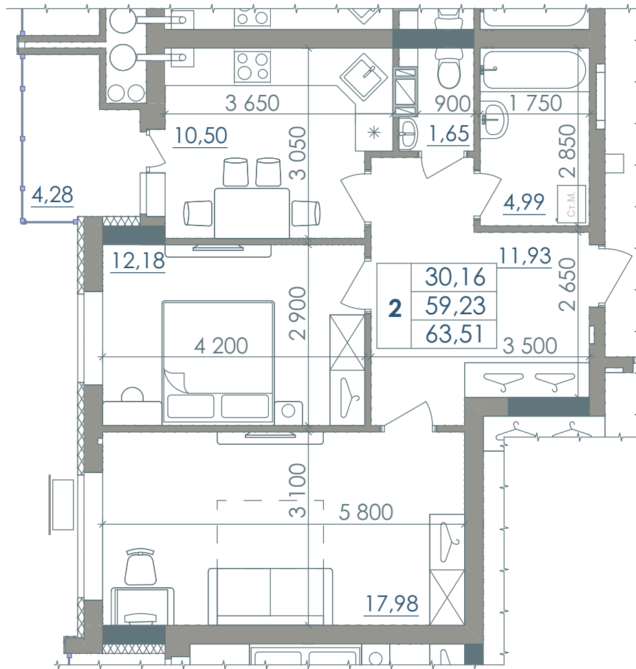
Графічне зображення схеми будівельного плану МОН - №166
