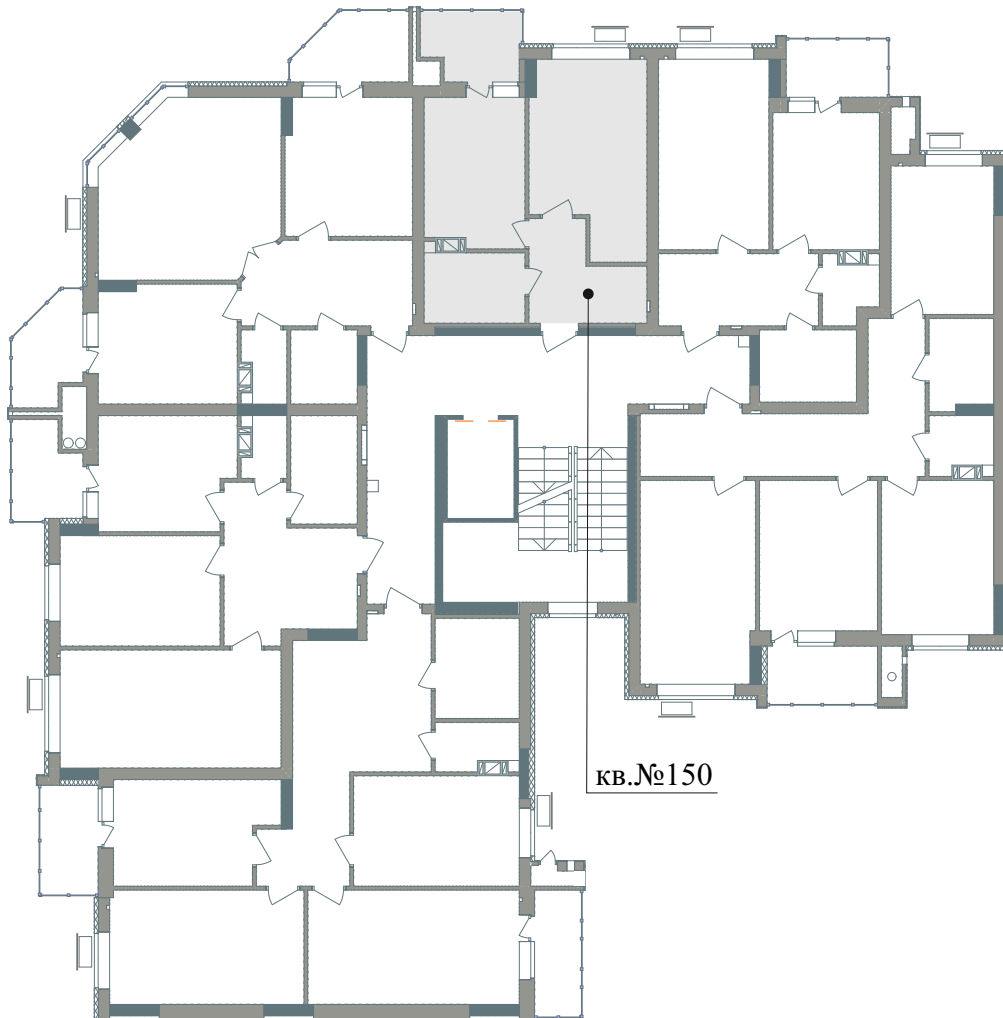
Схема розміщення МОН - №150 на поверсі
