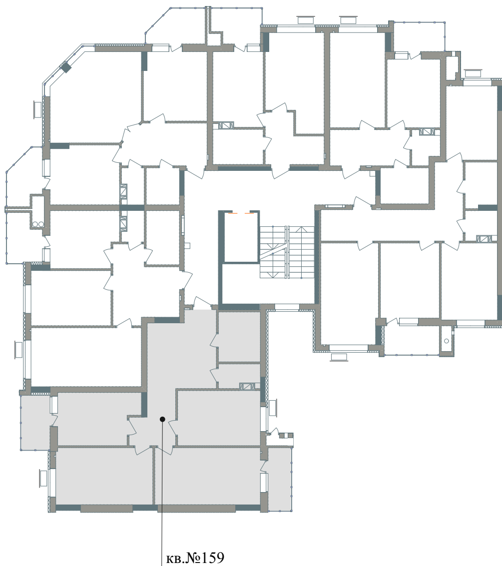
Схема розміщення МОН - №159 на поверсі
