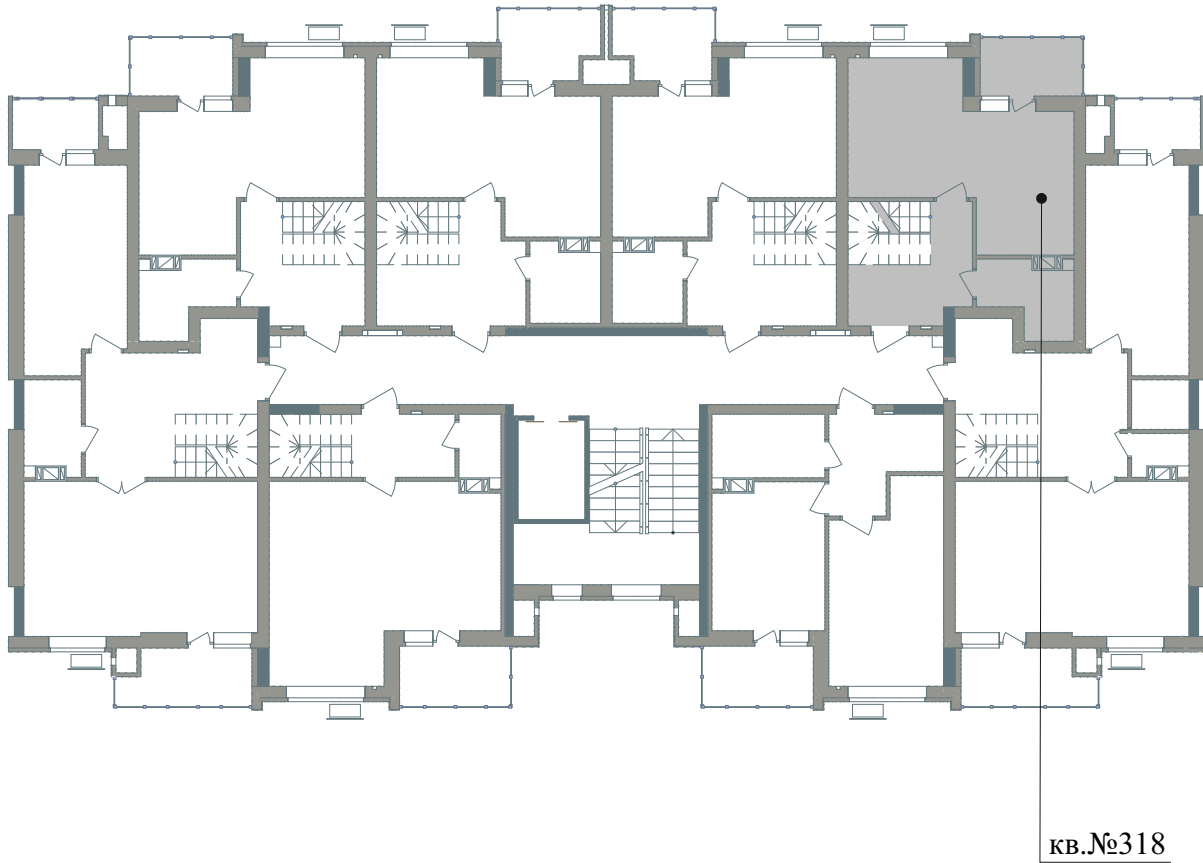
Схема розміщення МОН - №318 на поверсі
