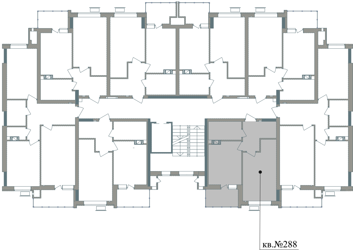
Схема розміщення МОН - №288 на поверсі
