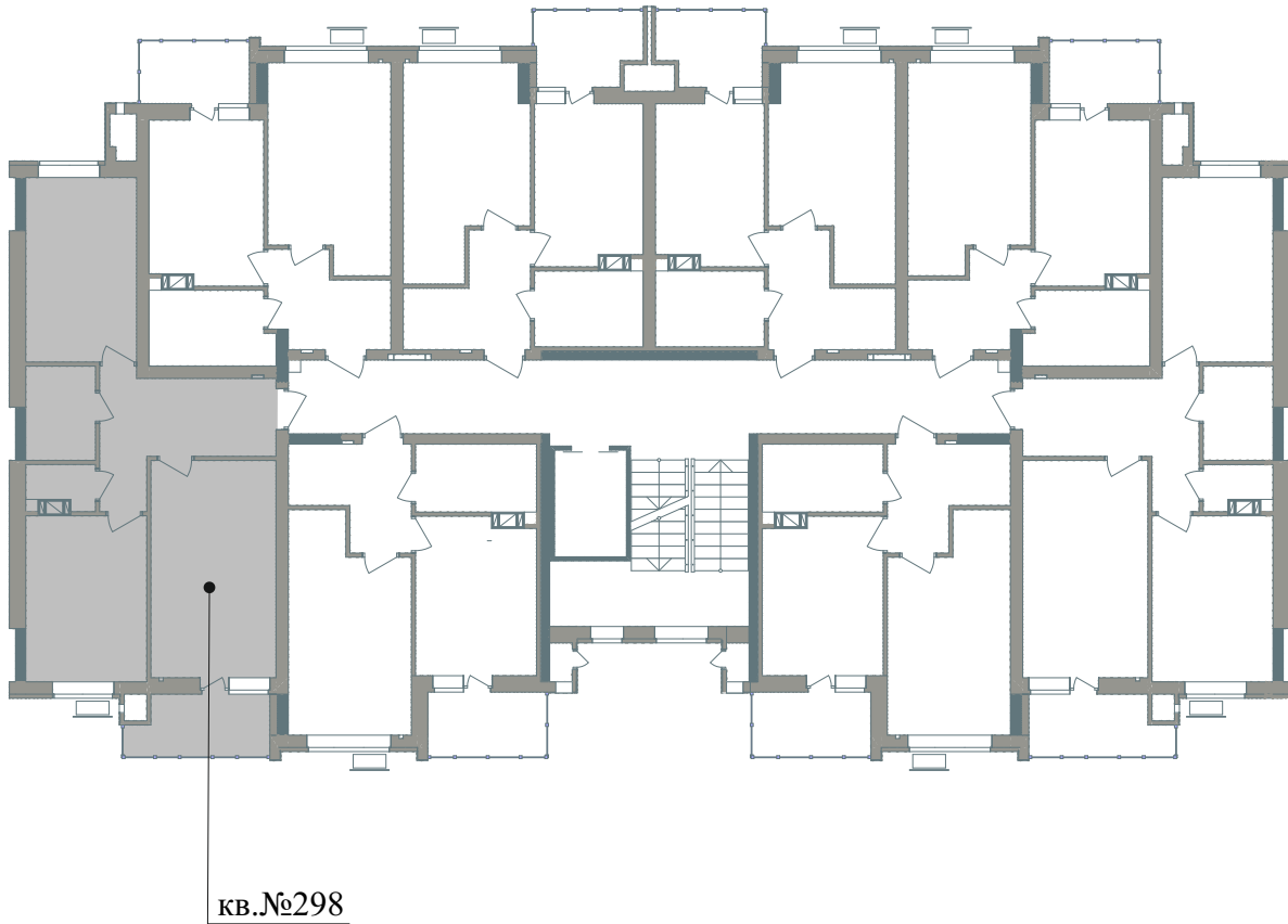
Схема розміщення МОН - №298 на поверсі
