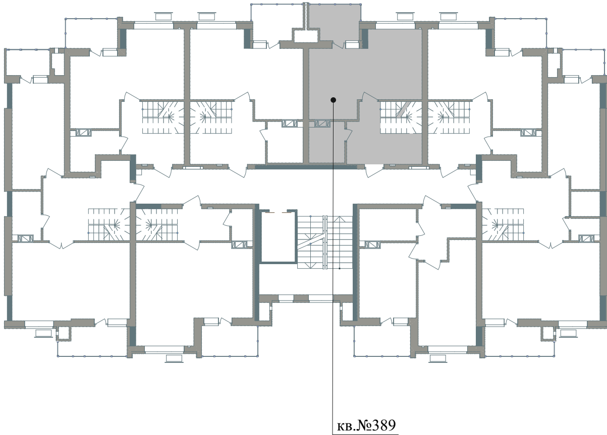
Схема розміщення МОН - №389 на поверсі
