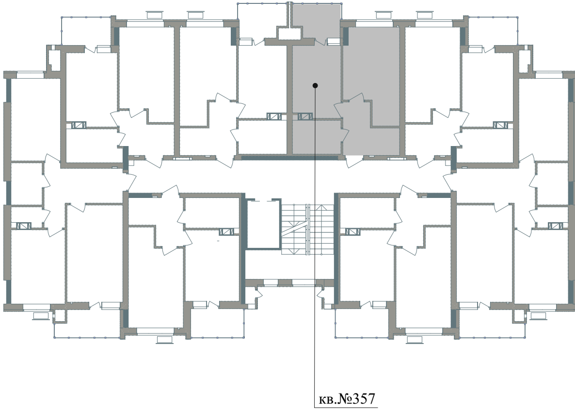
Схема розміщення МОН - №357 на поверсі
