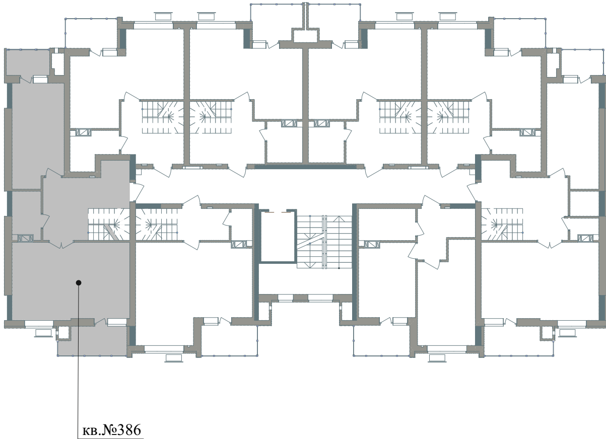
Схема розміщення МОН - №386 на поверсі
