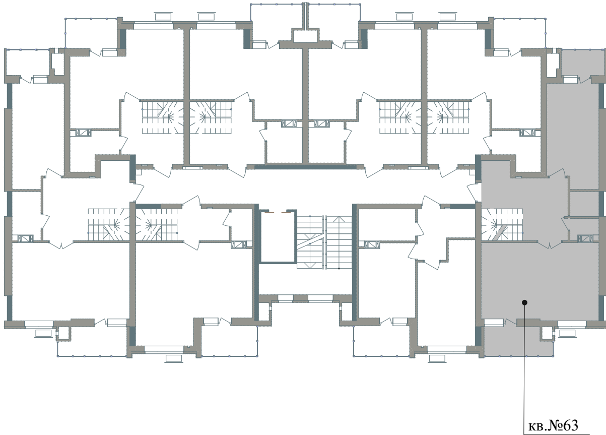
Схема розміщення МОН - №63 на поверсі
