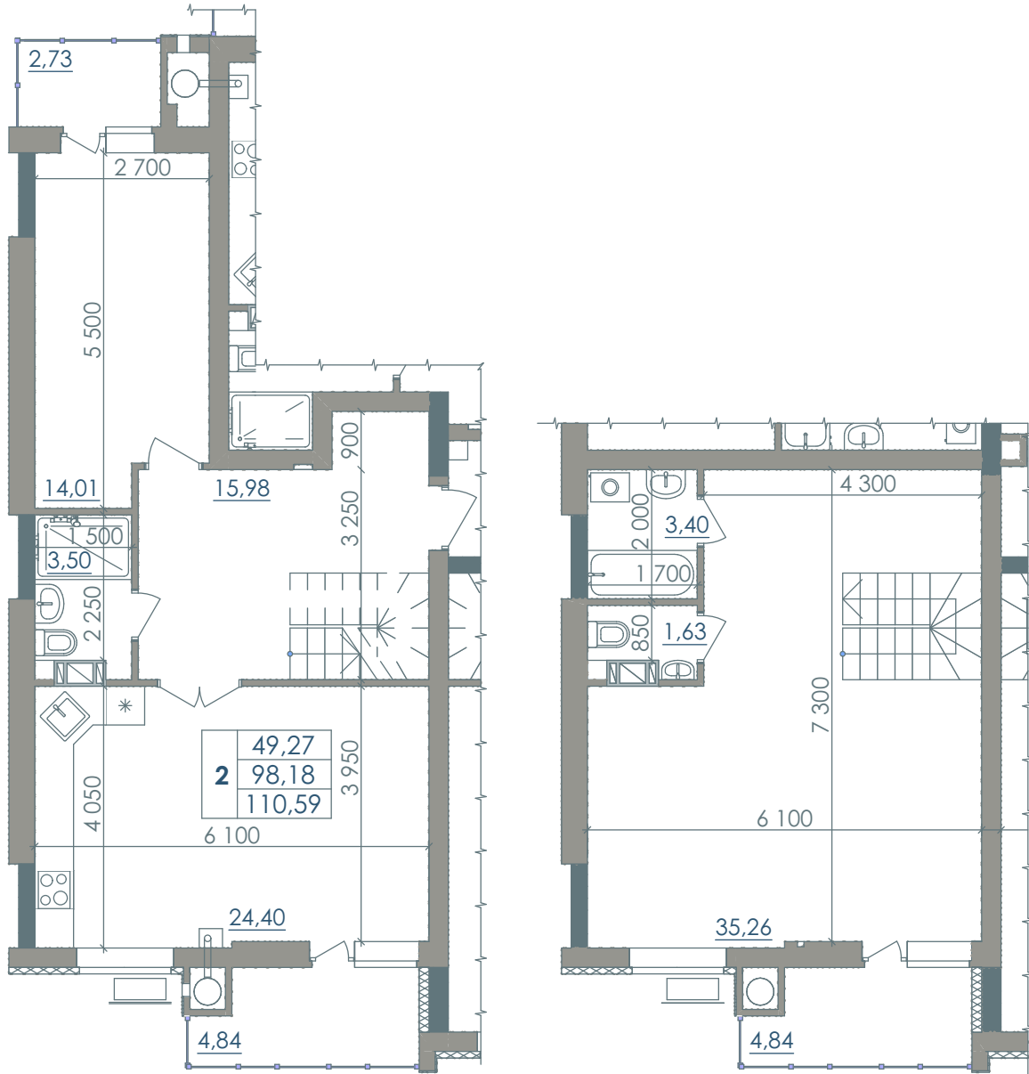
Графічне зображення схеми будівельного плану МОН - №58
