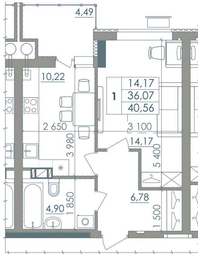
Графічне зображення схеми будівельного плану МОН - №53
